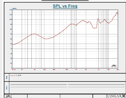
Графік АЧХ ВЧ
