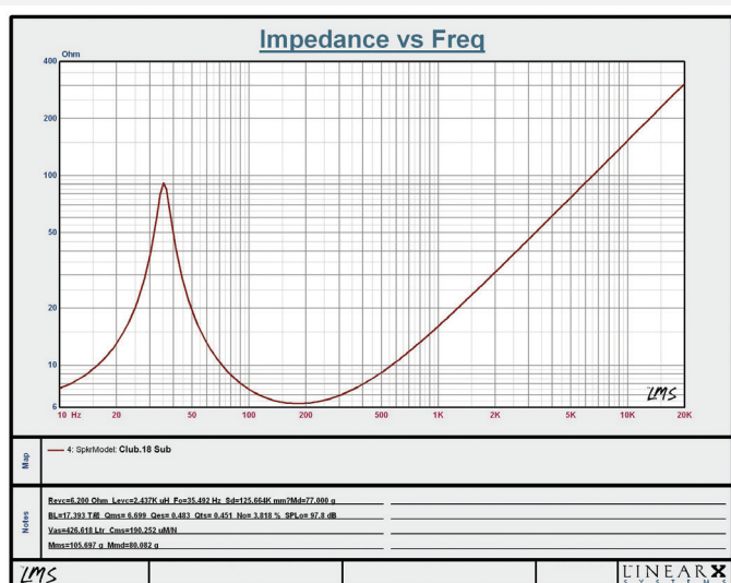
Графік АЧХ
