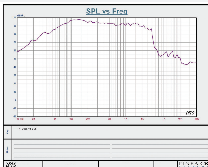
Графік АЧХ НЧ
